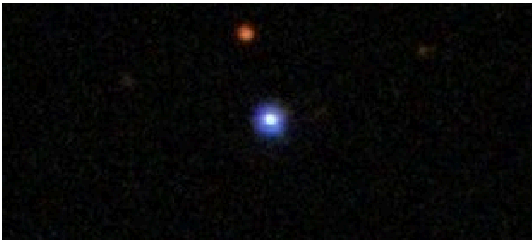
Imagen real de TON 618 (punto azul brillante)
